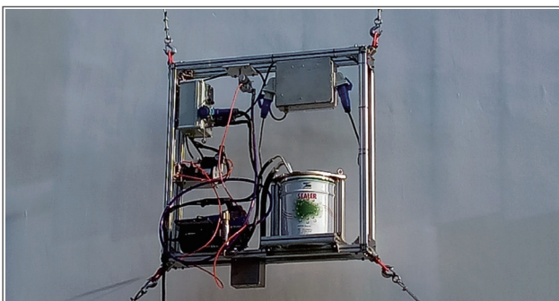
2018 香港工商業獎：設備及機器設計獎 - 奧馬迪機器人有限公司的鋼索機器人 2018 Hong Kong Awards for Industries: Equipment and Machinery Design Award - Cable Robot by O/Matic Intelligent Robot Limited
