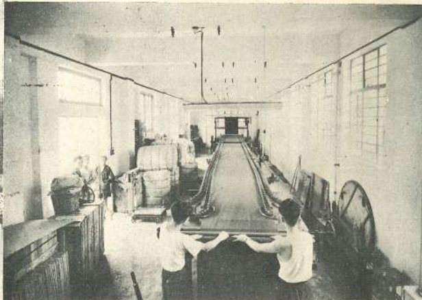
Sizing Machine 拉幅機
