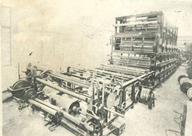
漿紗機
